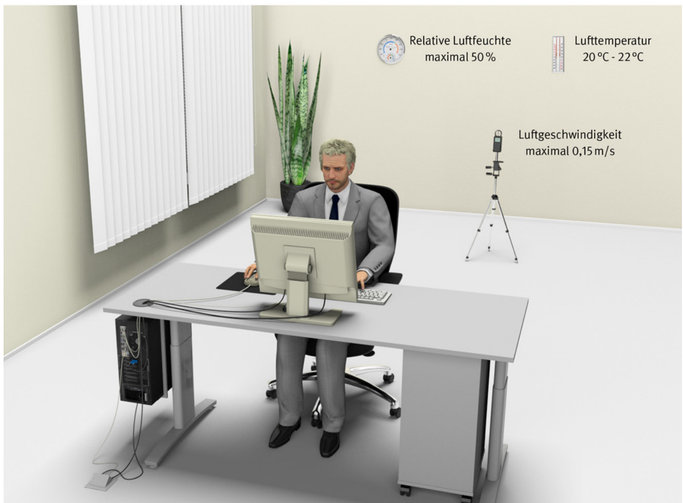
Abb. 47 Behaglichkeitsbereich
