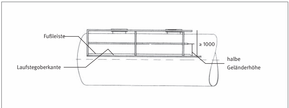
Laufsteg mit feststehendem Geländer
